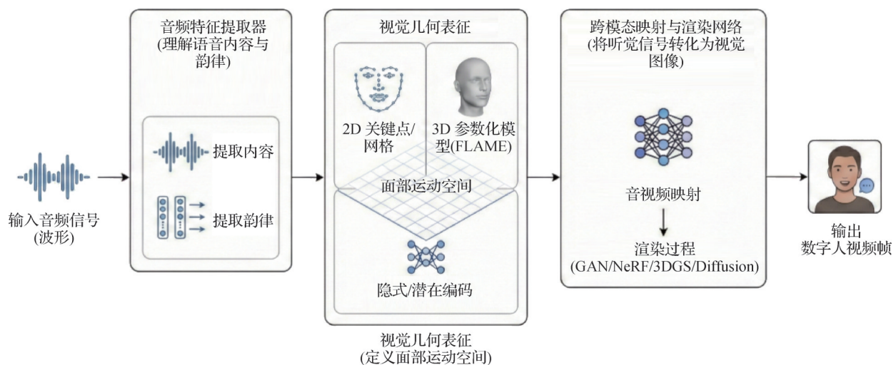
图1 音频驱动数字人的通用框架
